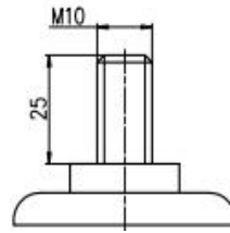
丝杆
