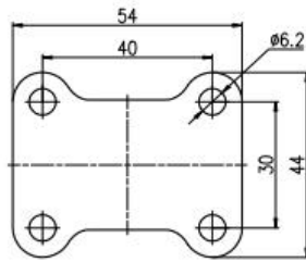
平板定向
